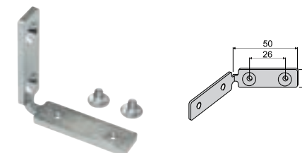
Kątownik montażowy GOLA
